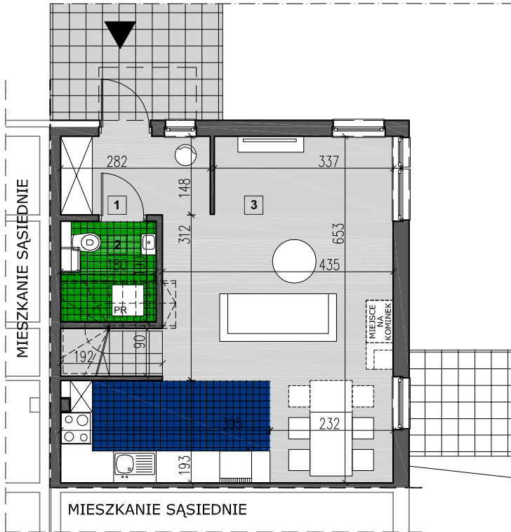
RZUT PARTERU
