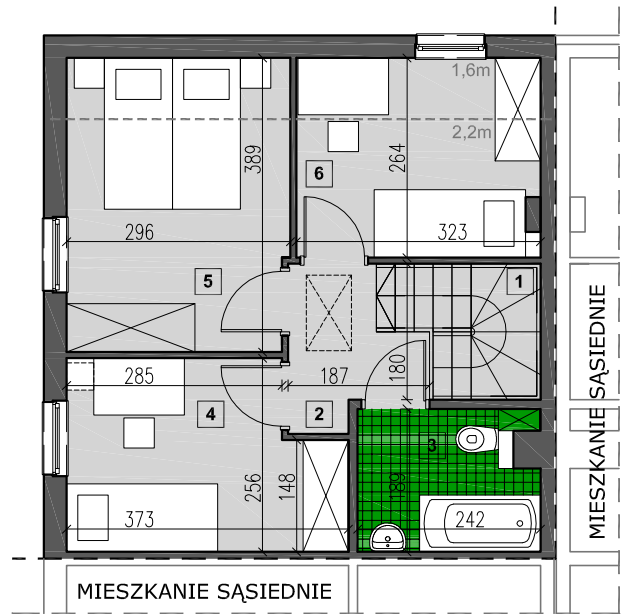
RZUT PIĘTRA
