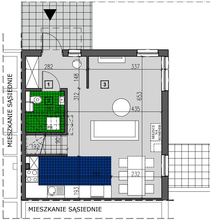
RZUT PARTERU
