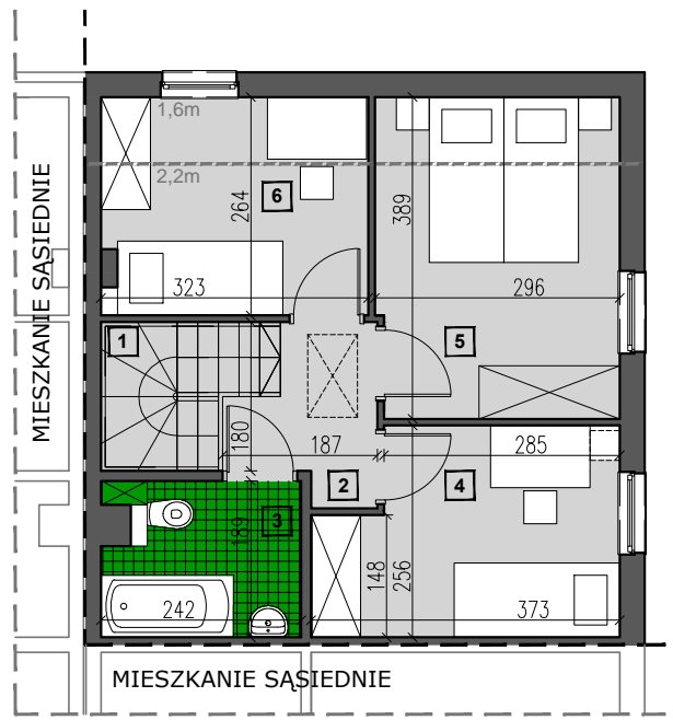
RZUT PIĘTRA
